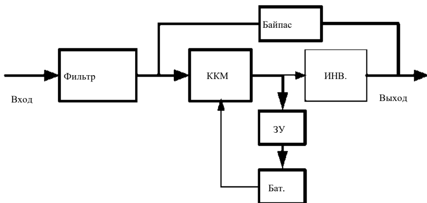
Рисунок 4.2 – Режим байпаса
