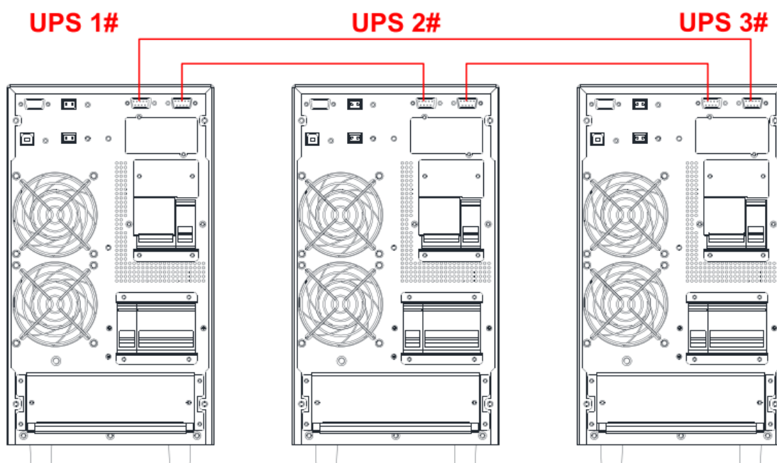
Рисунок 6.4 – Три параллельные системы ИБП
