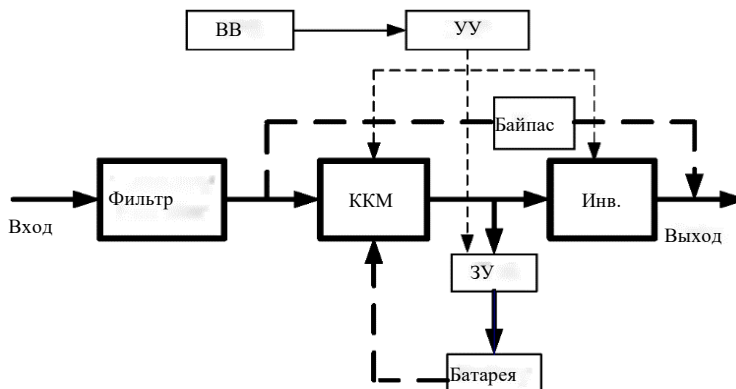
Рисунок 3 – Система ИБП
