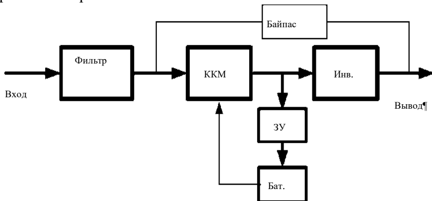
Рисунок 4.1 – Обычный режим
