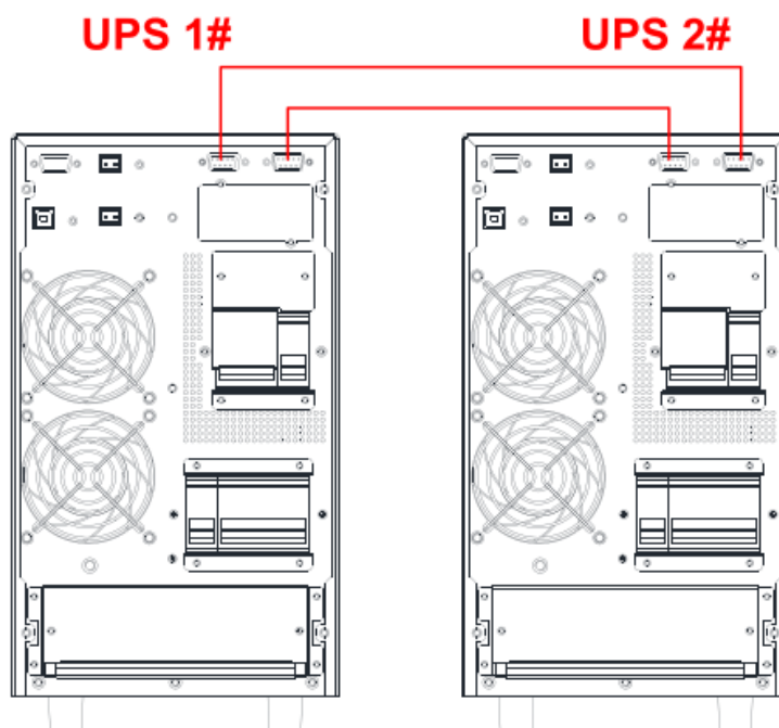
Рисунок 6.3 – Две параллельные системы ИБП
