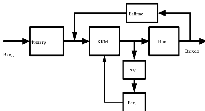
Рисунок 4.5 – Режим самотестирования
