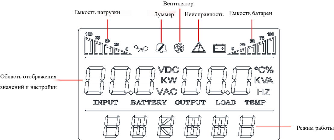
Рисунок 7.2 – Меню ЖК-дисплея
