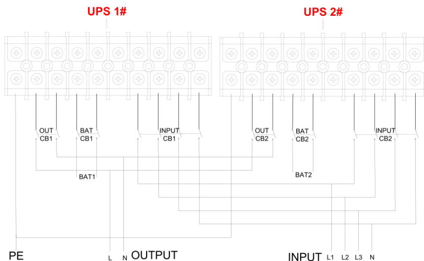
Рисунок 6.2 – Схема параллельной проводки
