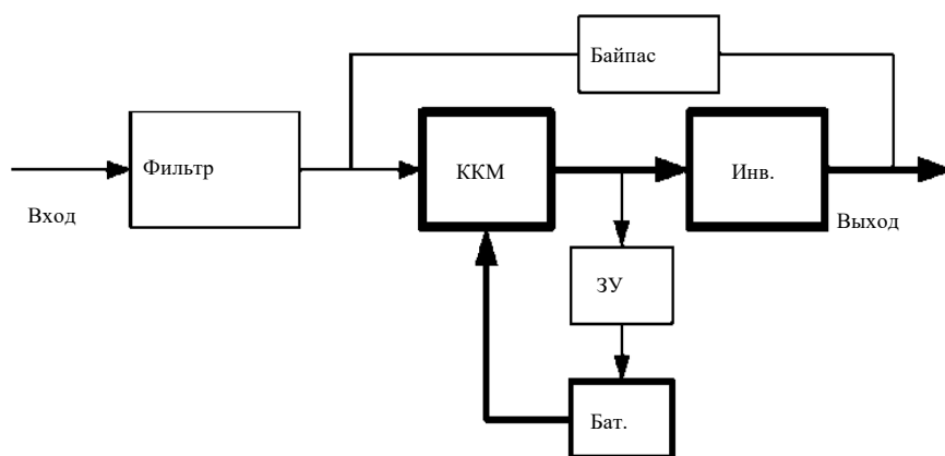
Рисунок 4.3 – Режим работы от батареи
