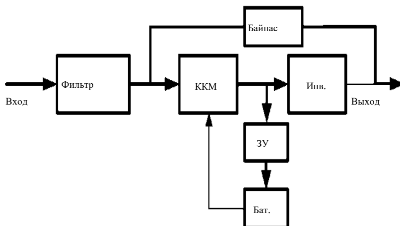
Рисунок 4.4 – Режим ЕСО
