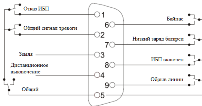
Рисунок 9.4 – Схема карты сухих контактов
