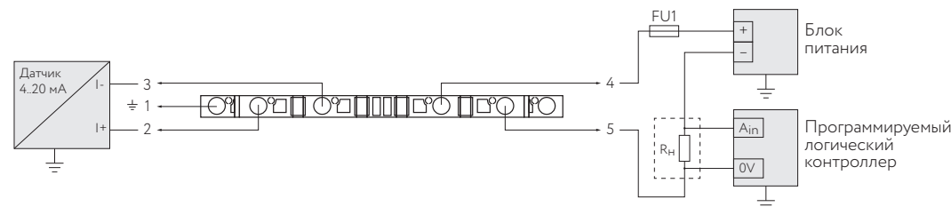
Рисунок 5. Схема применения УЗИП
